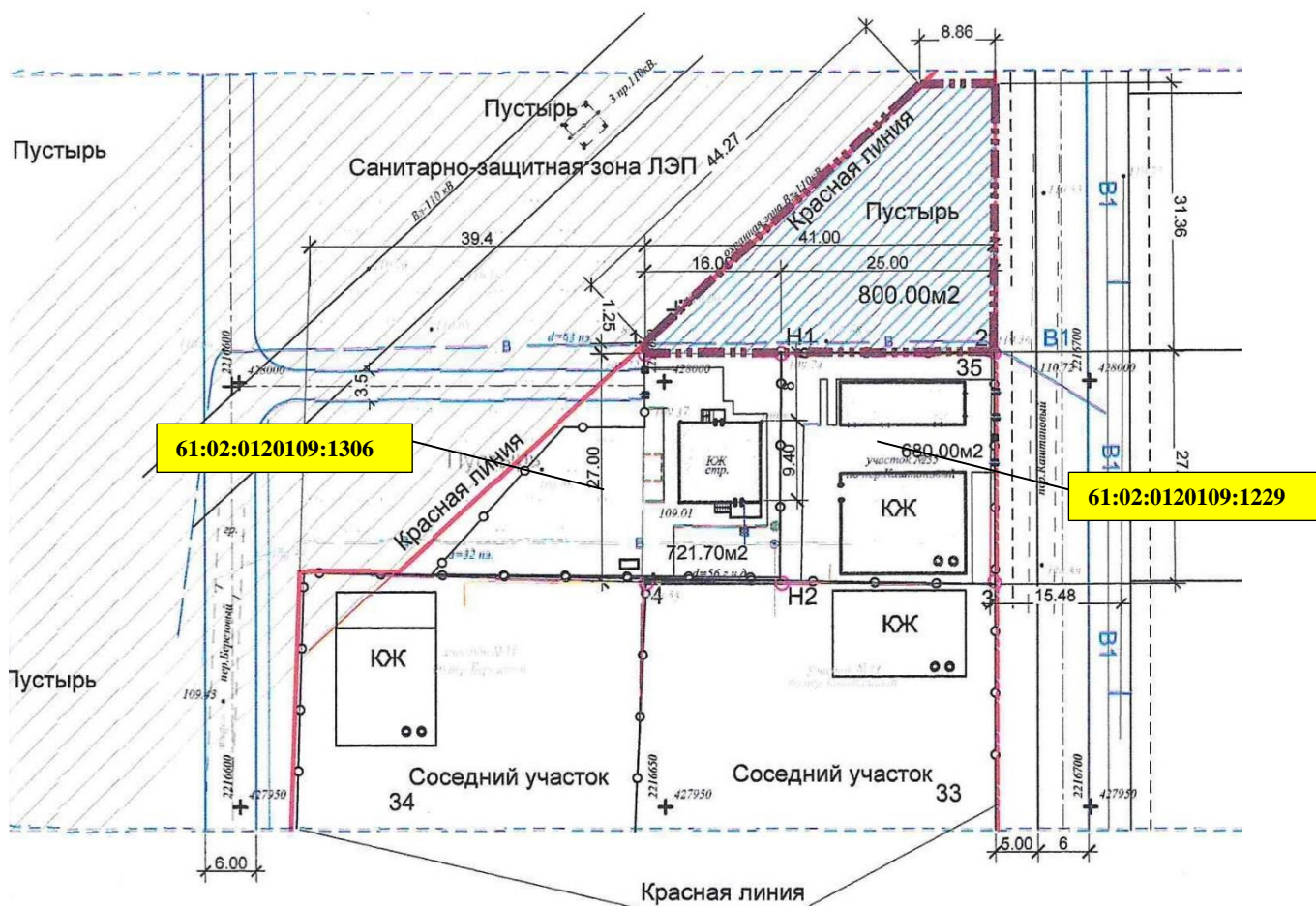
Схема планировочной организации земельного участка.
