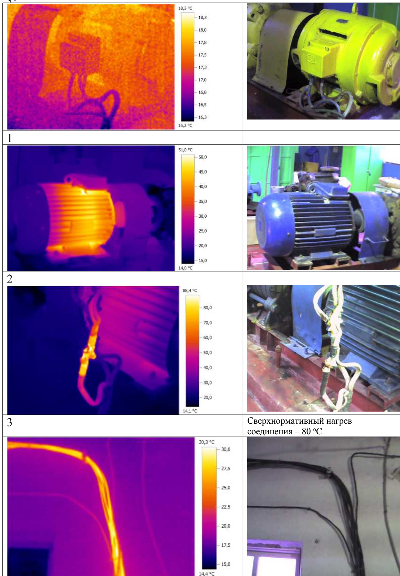
Рисунок 13 Тепловизионное (термографическое) обследование объектов ЦСХПВ
