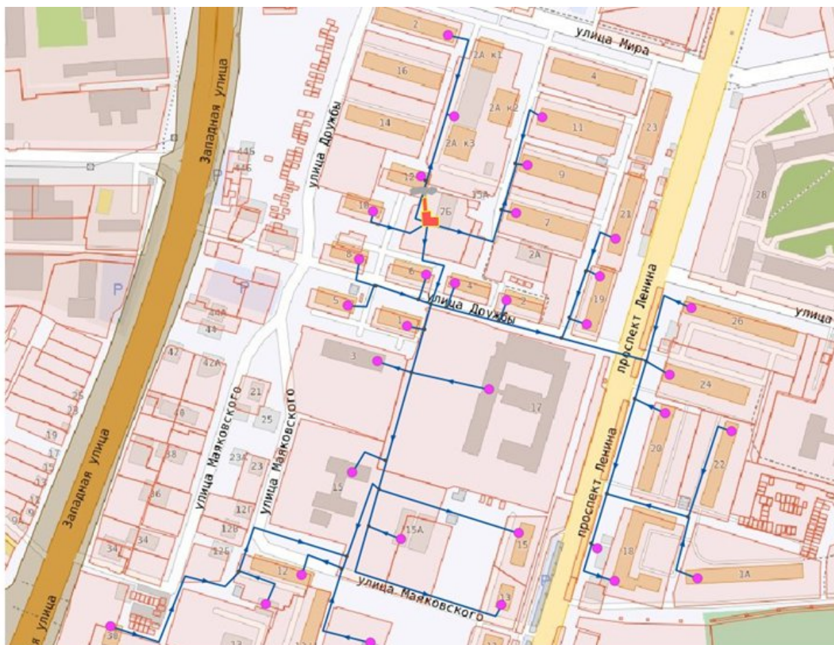
Рисунок 20 Схема теплоснабжения котельной № 3
