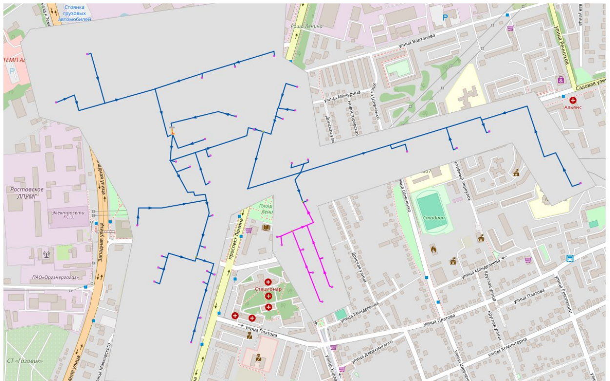
Рисунок 19 Схема теплоснабжения котельной № 1
