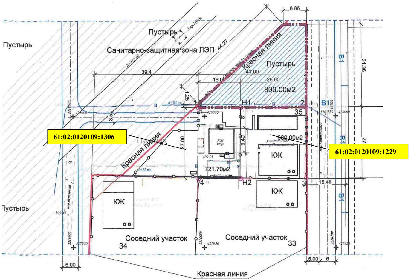
Схема планировочной организации земельного участка.
